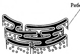
Эндоплазматическая сеть
