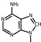
Аденин (A)
